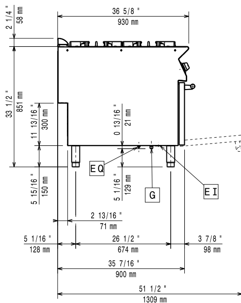
Zij aanzicht
